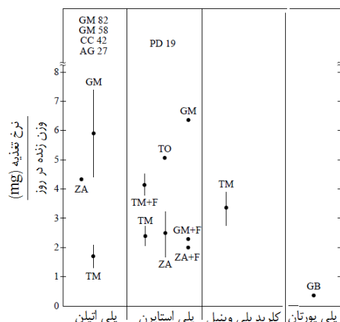
AG = لارو پروانه موم خوار ( Achroia grisella ) PD = لارو سوسک ( Plesiophthalmus davidis ) CC = لارو پروانه برگخوار ( Corcyra cephalonica ) TM = لارو سوسک زرد آرد ( Tenebrio molitor ) GB = حشره کامل جیرجیرک ( Gryllus bimaculatus ) TO = لارو سوسک سیاه آرد ( Tenebrio obscurus ) GM = لارو پروانه موم خوار ( Galleria mellonella ) ZA = لارو سوسک میلوم ( Zophobas atratus )
